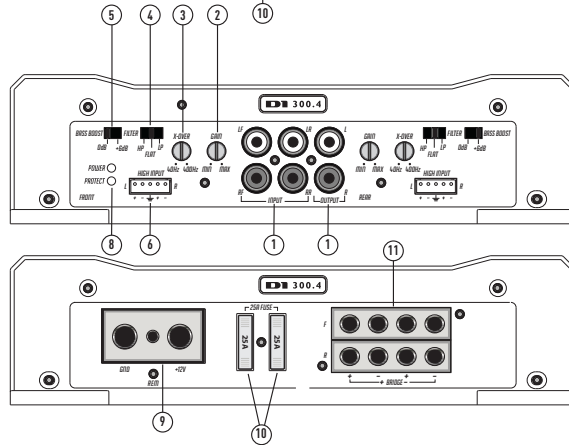
D1 300.4 4-Channel Amplifier
